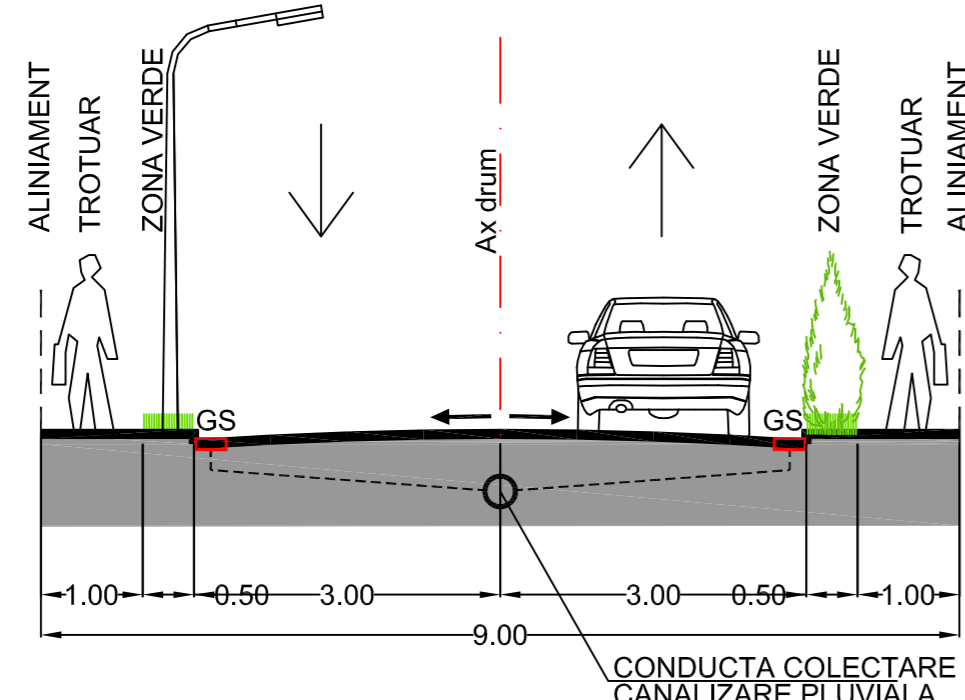
STRADA DE CATEGORIA A III-A - PROFIL TRANSVERSAL P1-P1, CU 2 BENZI DE CIRCULATIE
